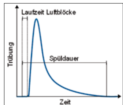
Abb. 2: Prinzipieller Trübungsverlauf während der Complex-Reinigung
