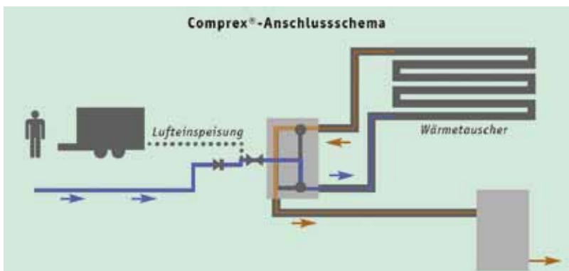
Abb. 7: Reinigen eines Wärmeübertragers mittels Complex-Verfahren über Umschaltstation
