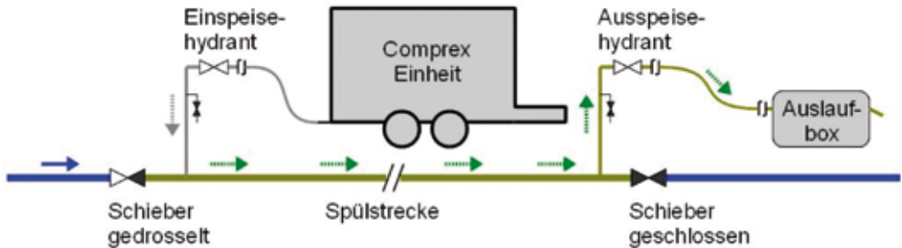
Abb. 4: Prinzip des Impuls-Spül-Verfahrens Comprex
