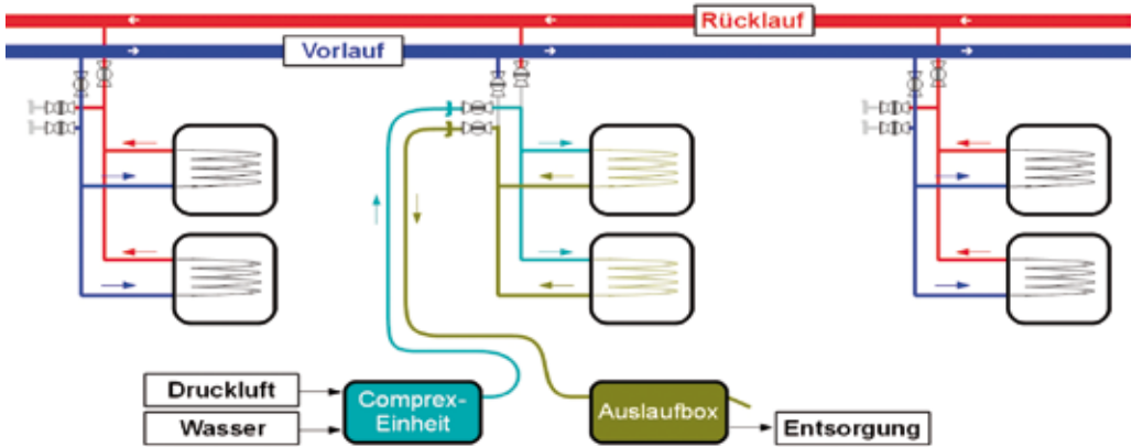
Abb. 3: Reinigung einer Gruppe im Kühlkreislauf mittels Comprex-Verfahren
