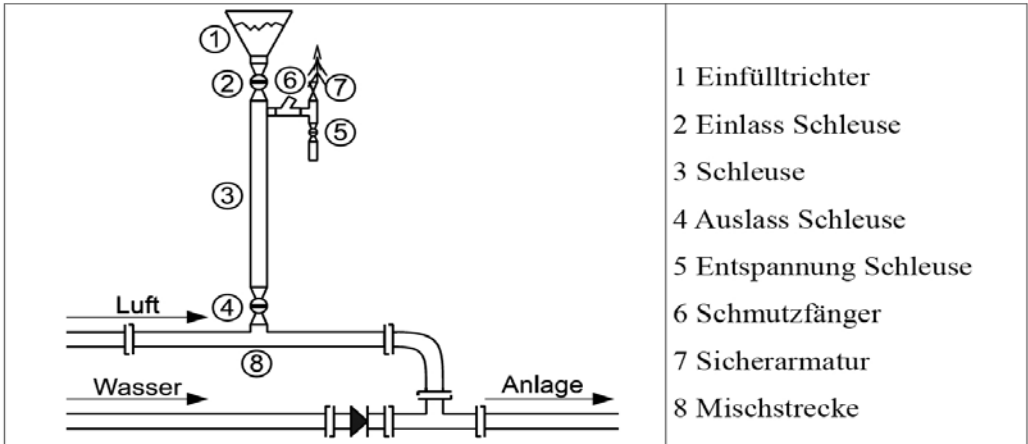
Abb. 8: Einheit zum Einbringen von Feststoffen (Feststoffinjektion) bei der Complex-Reinigung
