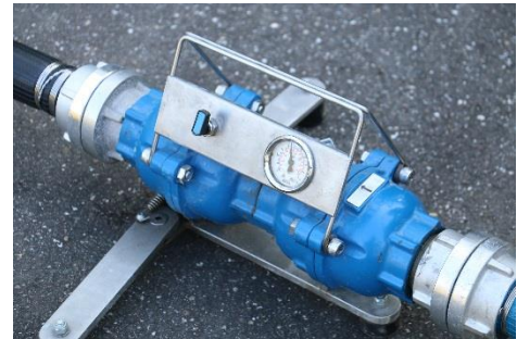
Abbildung 2: Hygieneschleuse
