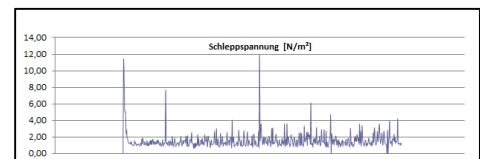
Abbildung 2: Beispiel für den Schleppspannungsverlauf während WSS
