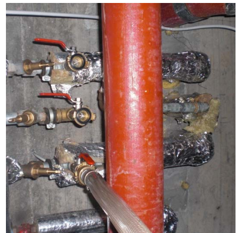
Abbildung 2: Einspeisung über Adapteranschlüsse
