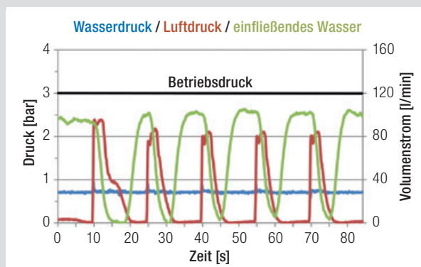
Abb. 2: Druck- und Volumenstromverlauf beim Impulsspülverfahren
