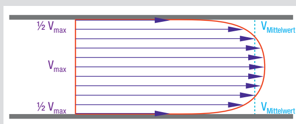
Abb. 1: Fließgeschwindigkeitsprofil bei turbulenter Strömung. Die Fließgeschwindigkeit ist dabei in der Mitte der Rohrleitung ( V_{max} ) doppelt so hoch wie an den Wandbereichen ( \frac{1}{2} V_{max} ).
